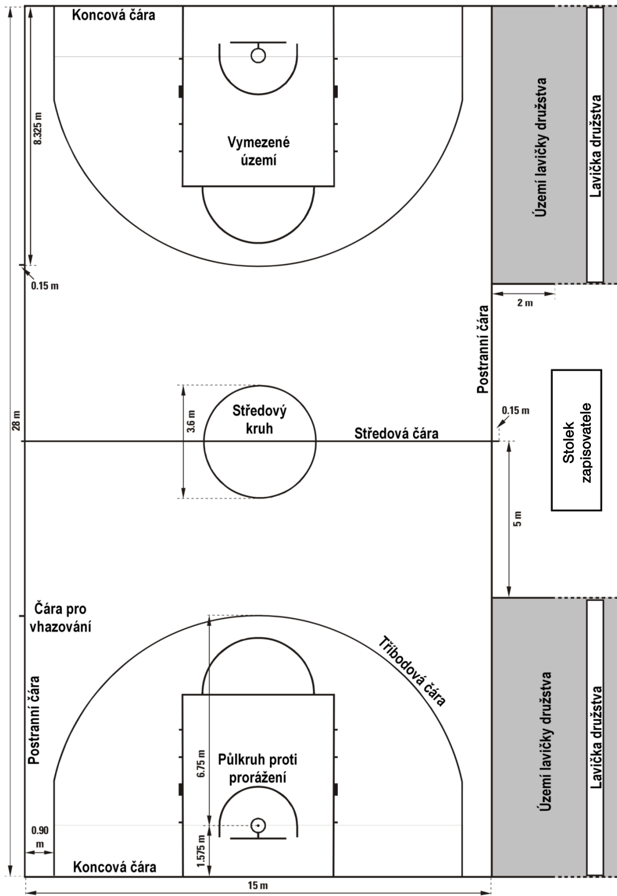
Obrázek 1 Rozměry hřiště
